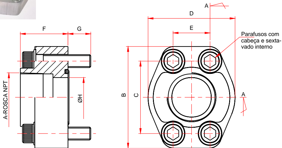
CORTE AA
